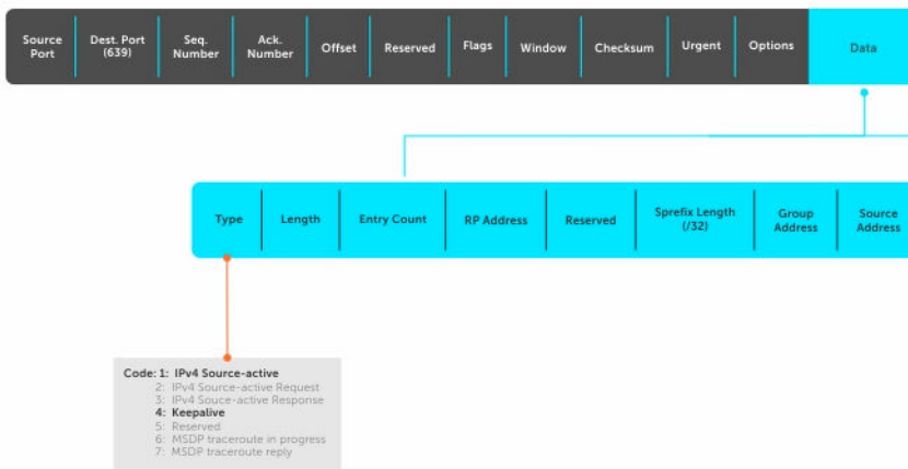
Figure 75. MSDP SA Message Format
